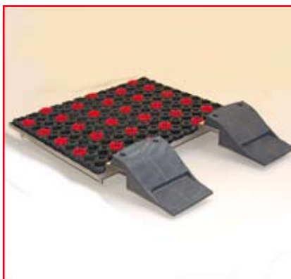
SHOT Open-Air Hack-Set mit Marco Hackschalen, Niveauegleichsmatte, 4 Eisverankerungs- dorne, 1 Ankerschraube als Niederhalterung, komplett mit Gummiwabenmatte und 30 eingesteckten Bürsten
